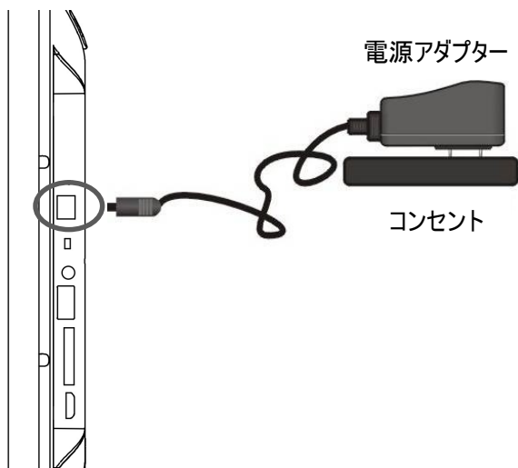
本体側面図
