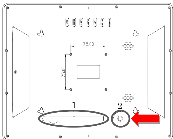
本体背面図
